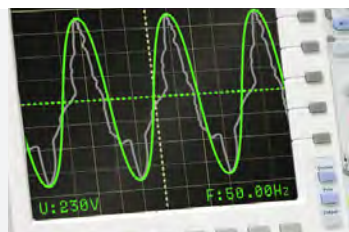
REINE SINUSWELLE
