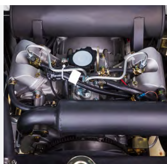
LEISTUNGSSTARKER ZWEIZYLINDER-MOTOR
